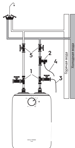
Рис. 4. Схема подключения к водопроводу моделей Terse U
