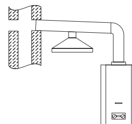
Рис. 14. Два устройства имеют одно подсоединение к дымоходу.
