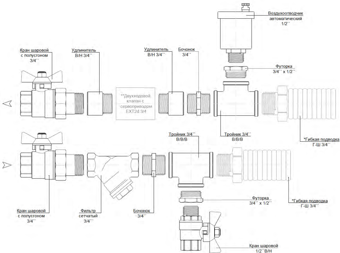
Рис. 2. Сантехнический комплект для обвязки 2С
