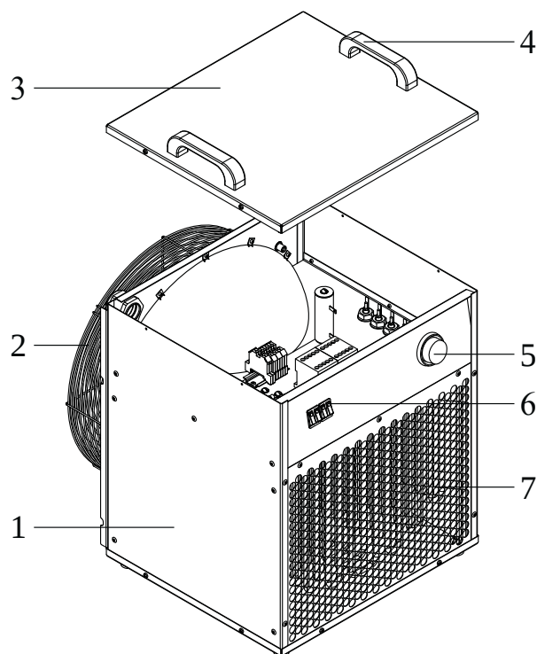
Рисунок 1. Тепловентилятор
