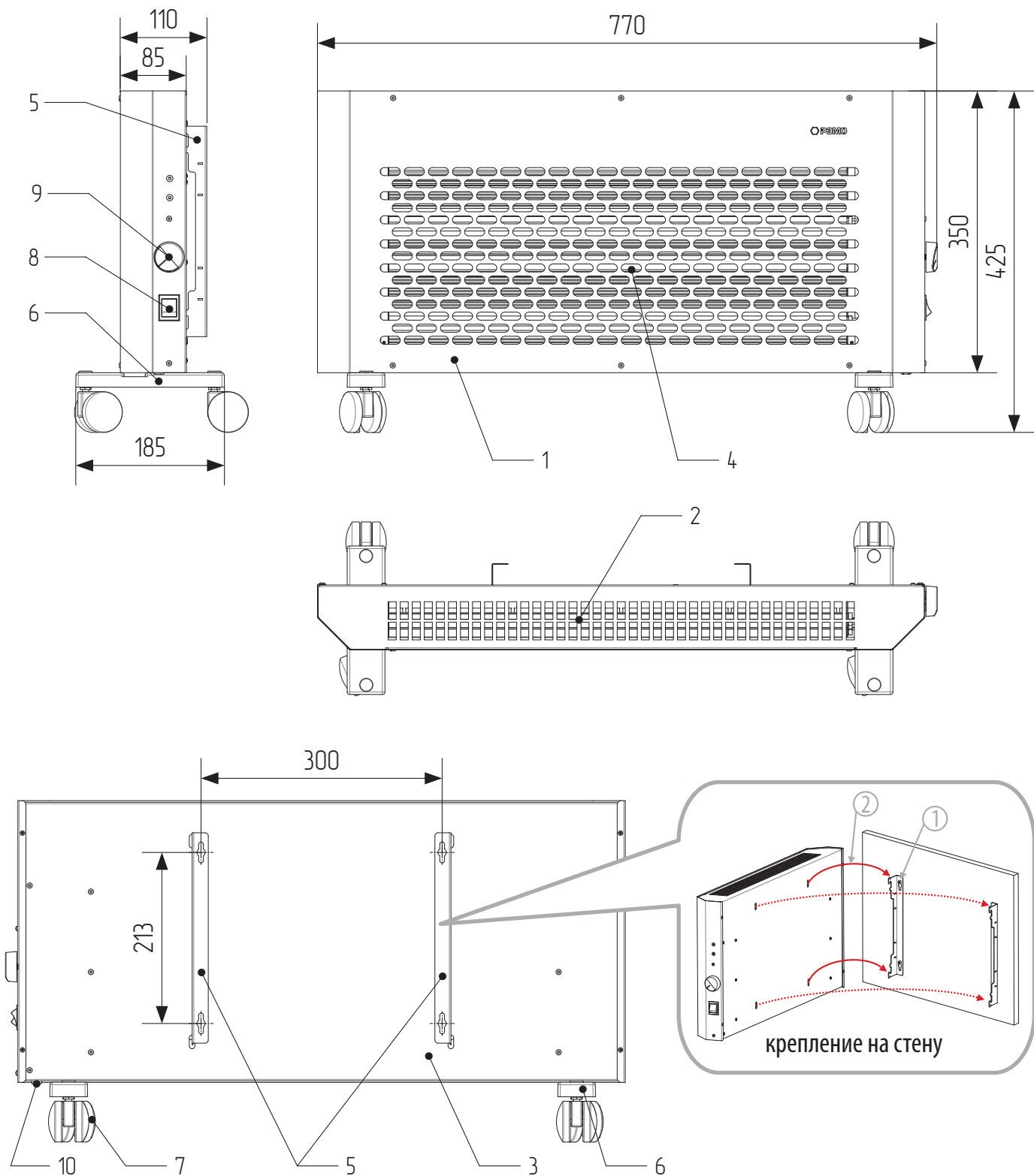
Рисунок 1. Габаритный чертёж и элементы конструкции электрического обогревателя.
