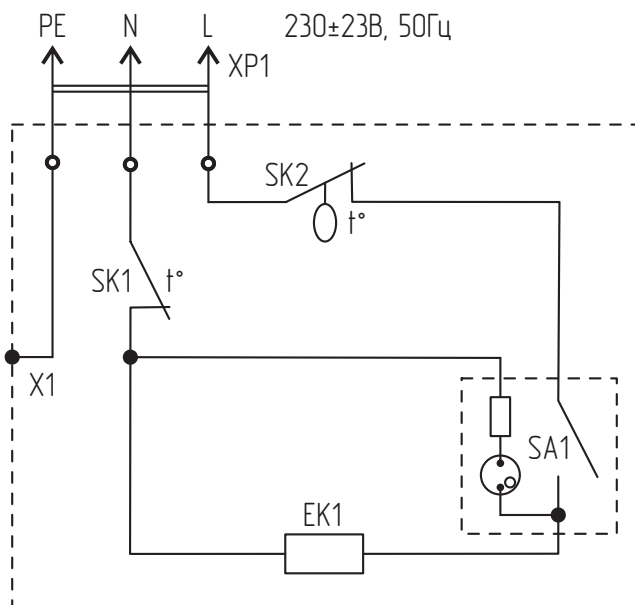
Рисунок 2. Электрическая схема конвектора
