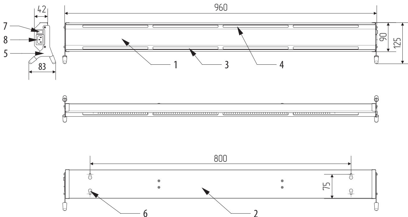
Рисунок 1. Габаритный чертёж и элементы конструкции электрического обогревателя.
