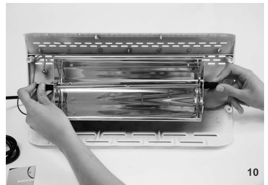
10. СОБЕРИТЕ ОБОГРЕВАТЕЛЬ, ПРОСЛЕДОВАВ СБОРКЕ В ОБРАТНОМ ПОРЯДКЕ.
