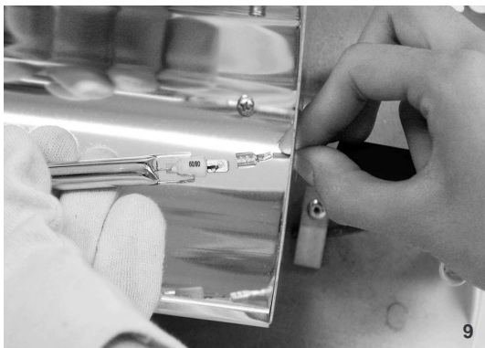
9. ПОДСОЕДИНИТЕ СОЕДИНИТЕЛЬНЫЕ РАЗЪЕМЫ НОВОЙ ЛАМПЫ ТИПА «ПАПА» К ДВУМ ПРОВОДАМ, НАТЯНИТЕ НА НИХ СИЛИКОНОВЫЕ КАПСУЛЫ И ВСТАВЬТЕ ЛАМПЫ НА ПРЕЖНЕЕ МЕСТО В МЕСТО РАСПОЖЕНИЯ ЗАЖИМОВ.
