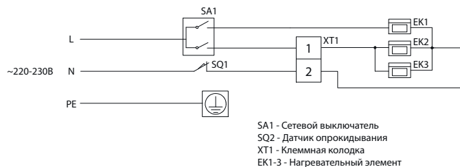
Рис. 1. Электрическая схема принципиальная BIGH-55 H
