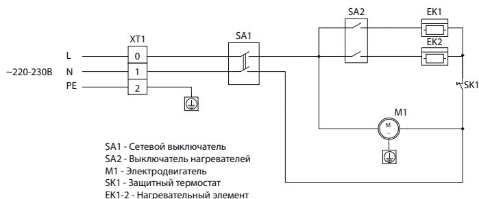
Рис. 2. Электрическая схема принципиальная BIGH-55 F
