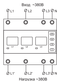
Рис.1. Схема подключения
