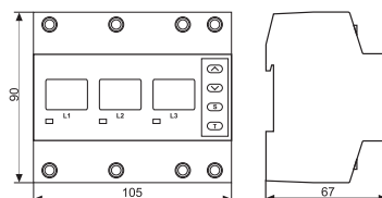
Рис.2. Габаритные размеры
