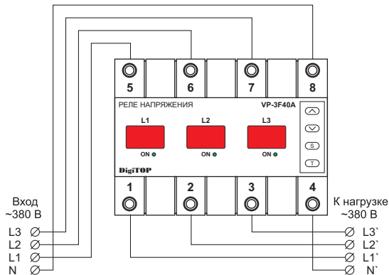
Схема подключения
